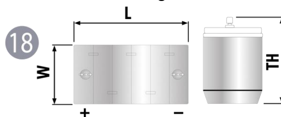
Terminal: Tornillo
