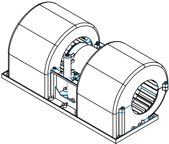
VISTA ISOMÉTRICA Isometric View Escala 1:5
