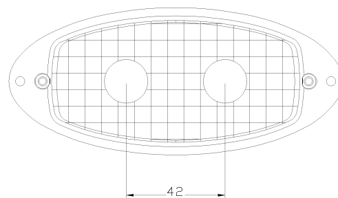
Vista frontal carcaça
