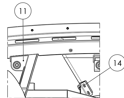
DETALHE "A" "A" DETAIL Scale 1:5
