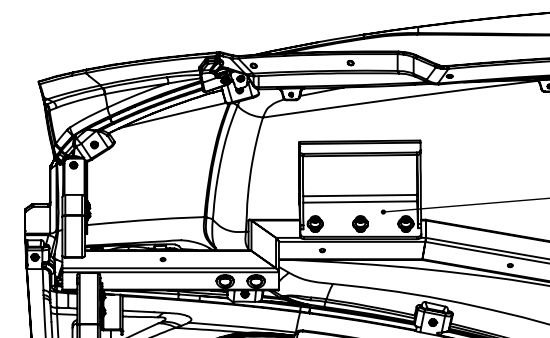
VISTA INFERIOR BOTTOM VIEW
