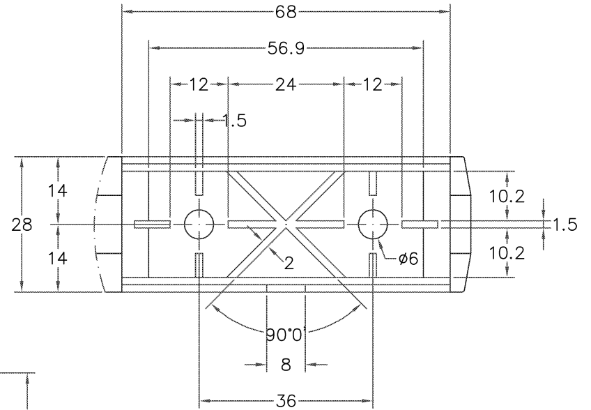
DETALHE "A" "A" DETAIL Scale 2:1.5
