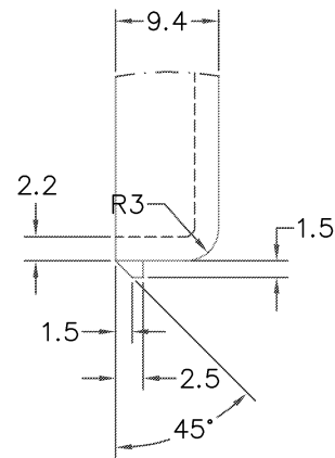
DETALHE "X"
