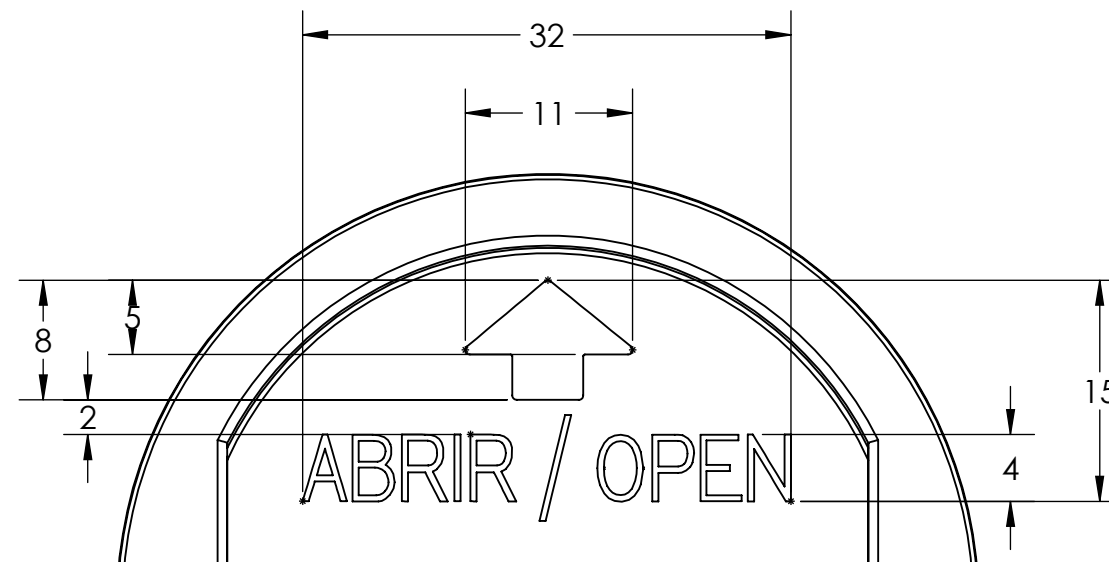
DETALHE "A" "A" DETAIL Scale 2:1
