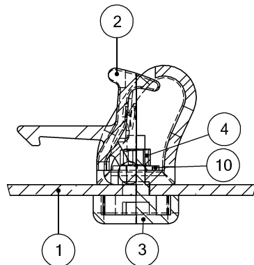
DETALHE "A" "A" DETAIL Scale 1:1
