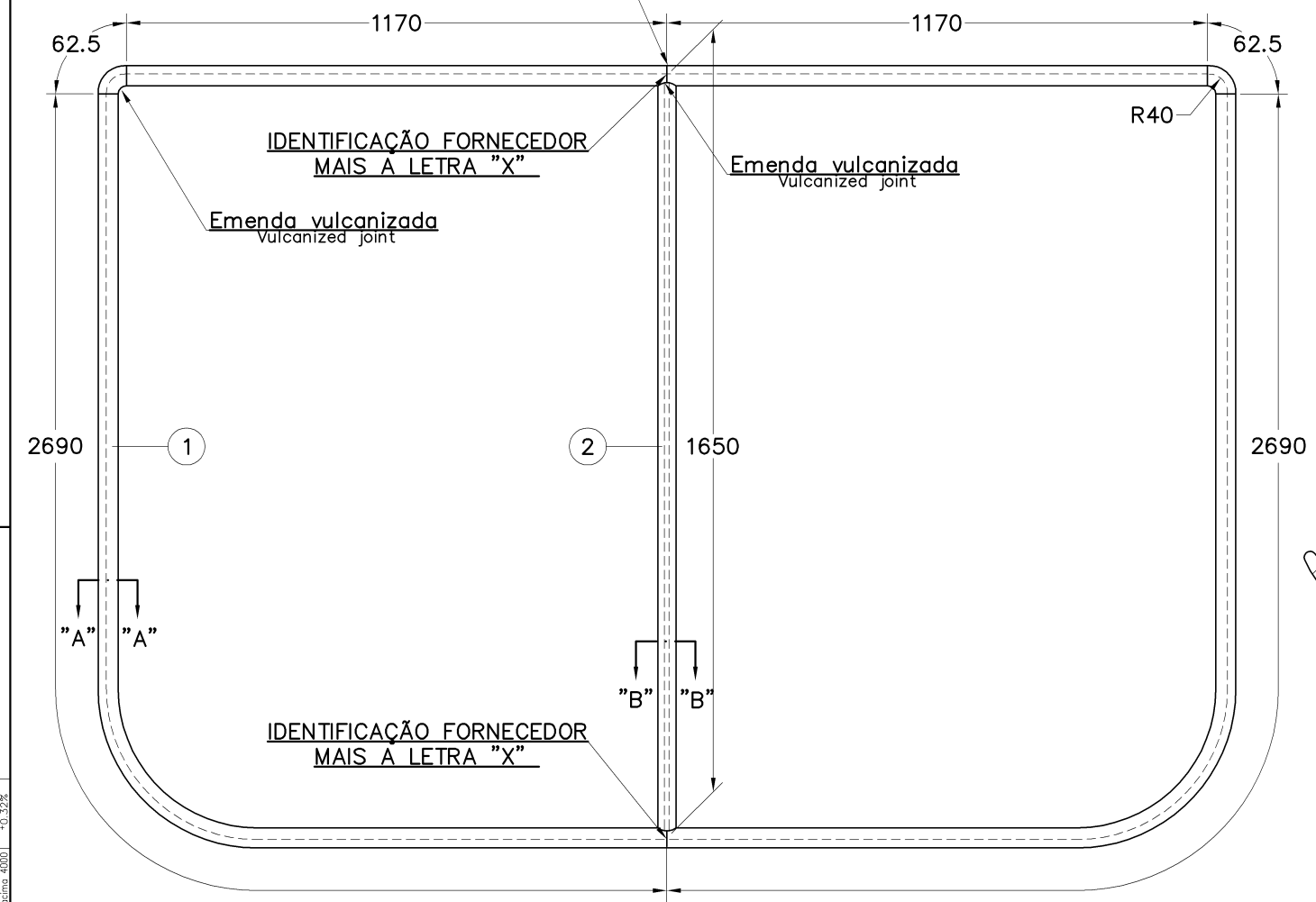
Referencia para dimensões Reference for dimensions SECCAO "AA" "AA" SECTION Scale 1:1
