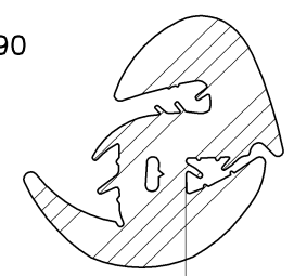
Referencia para dimensões Reference for dimensions SECCAO "AA" "AA" SECTION Scale 1:1
