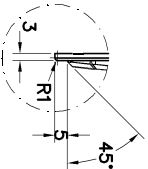
DETALHE "X" "X" DETAIL
