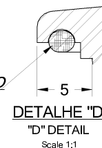
APLICAR PU PARA VEDAÇÃO APPLY PU TO SEALING
