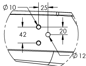
DETALHE "A"
