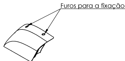
VISTA ISOMÉTRICA ISOMETRIC VIEW ESCALA 1:5
