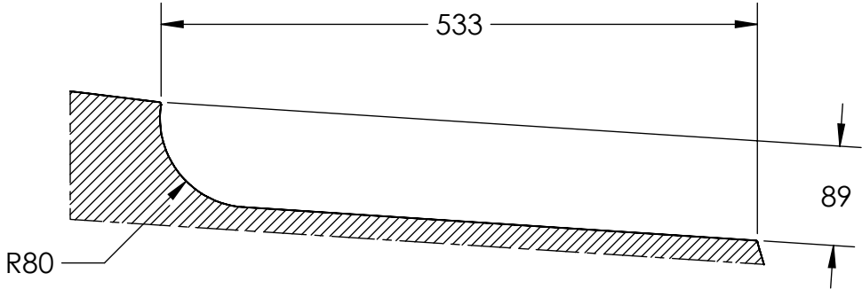
DETALHE "A" "A" DETAIL Scale 1:6
