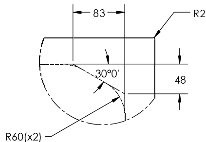
DETALHE "A"
