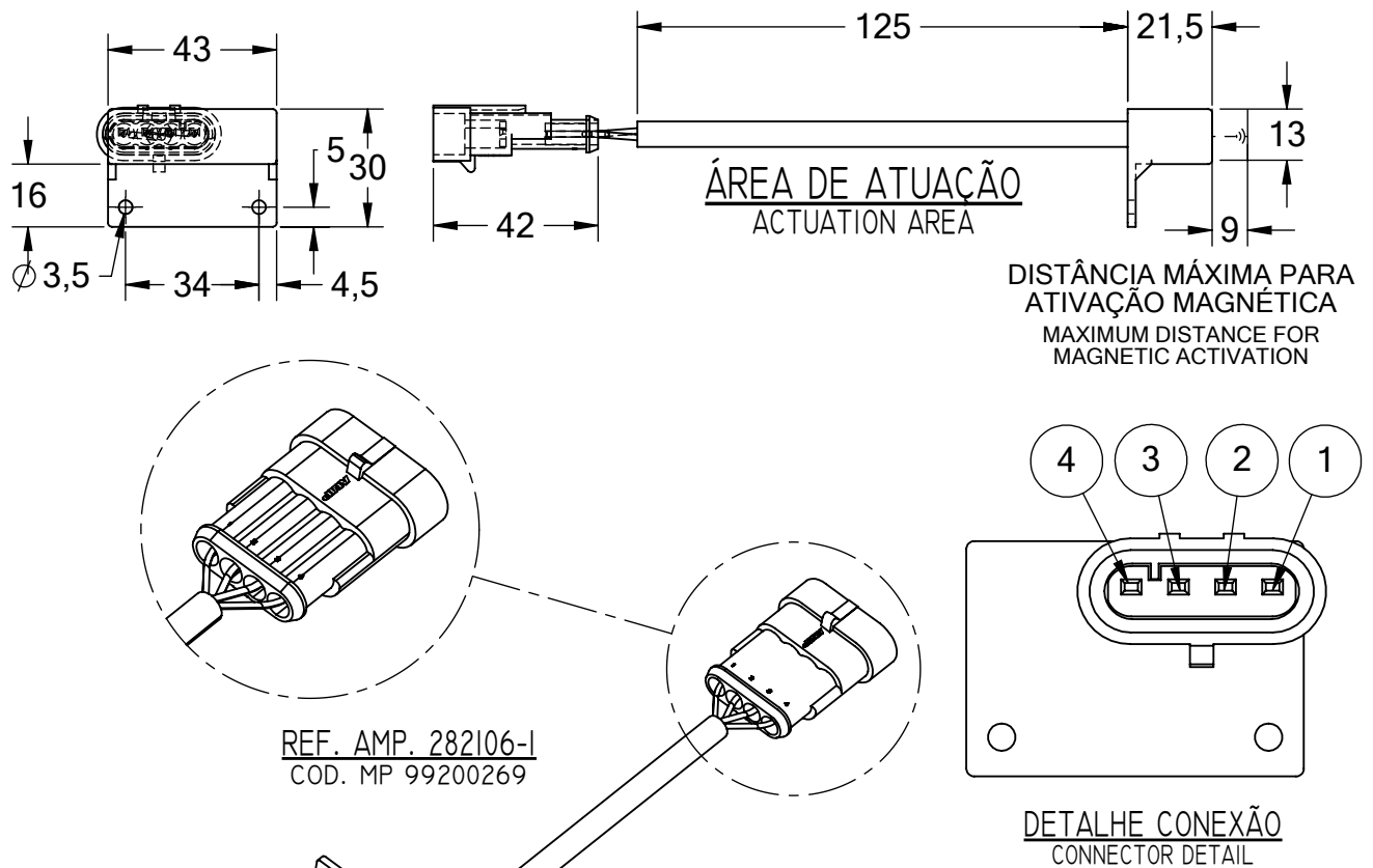
Diagrama funcional
