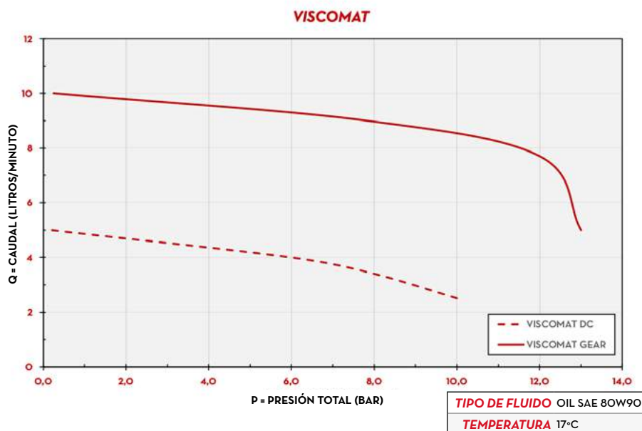
BOMBA DE ENGRANAJES
